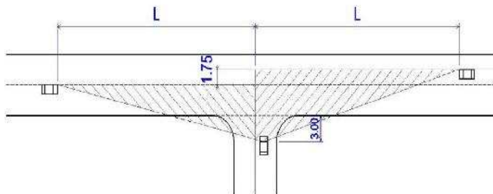
Uzbraukšanas un tuvošanās redzamības brīvlauku pleca garumi (L)
