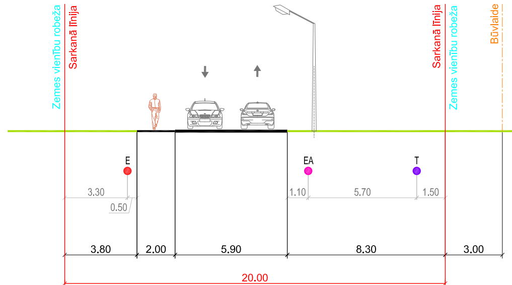
Šķēršprofils 1-1 (esošā situācija)
