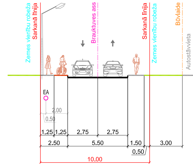
Šķēršprofils 2-2 (plānotā situācija)
