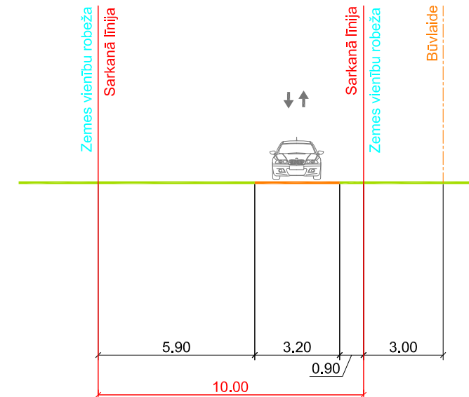
Šķēršprofils 2-2 (esošā situācija)
