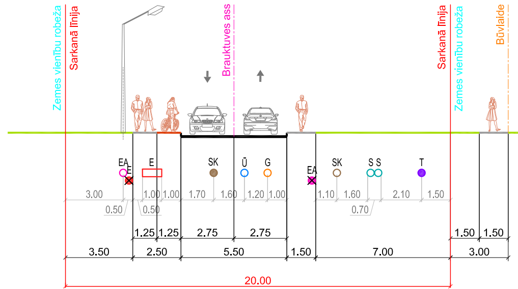
Šķēršprofils 1-1 (plānotā situācija)
